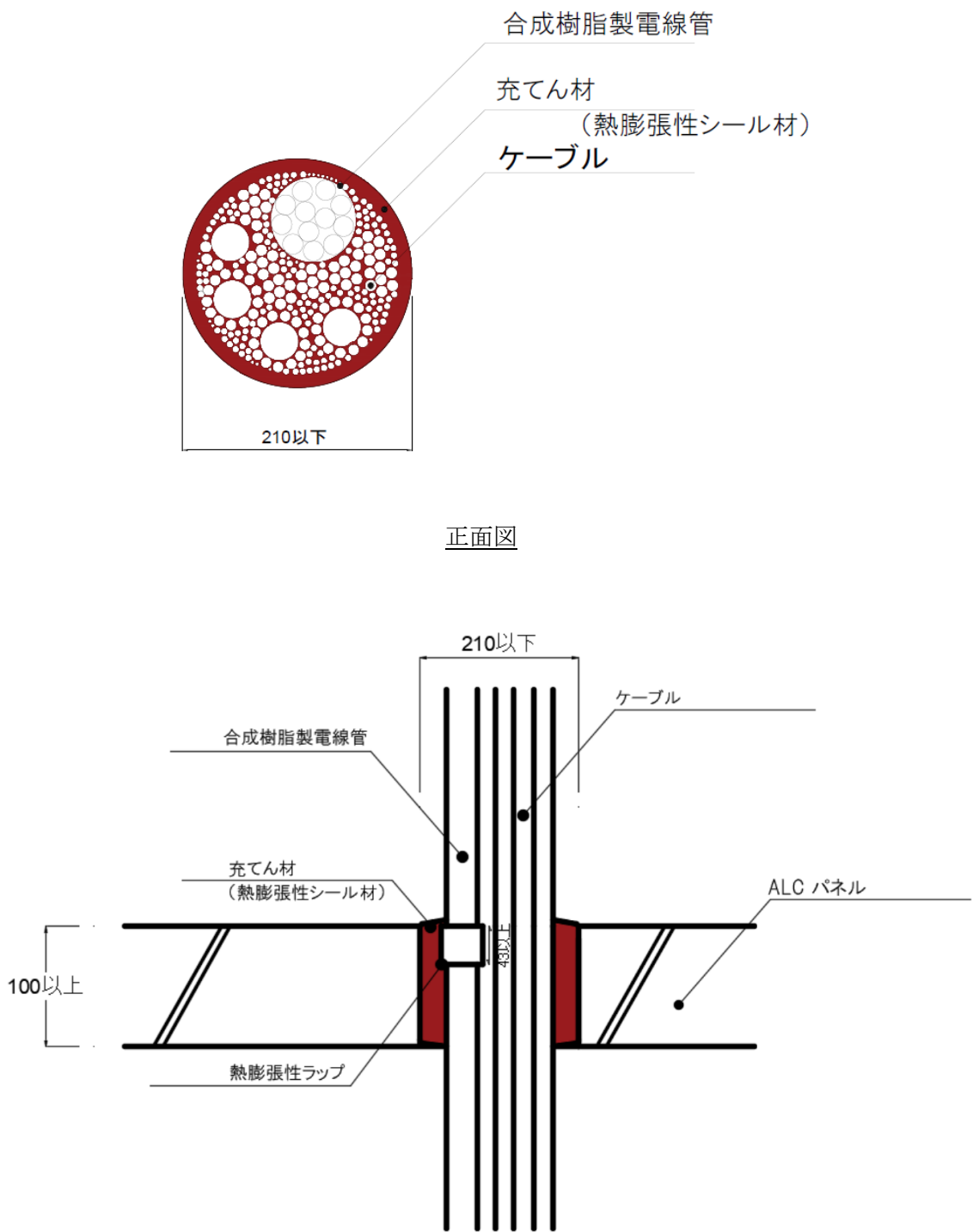
断面図 1 (スラブ上より施工)
