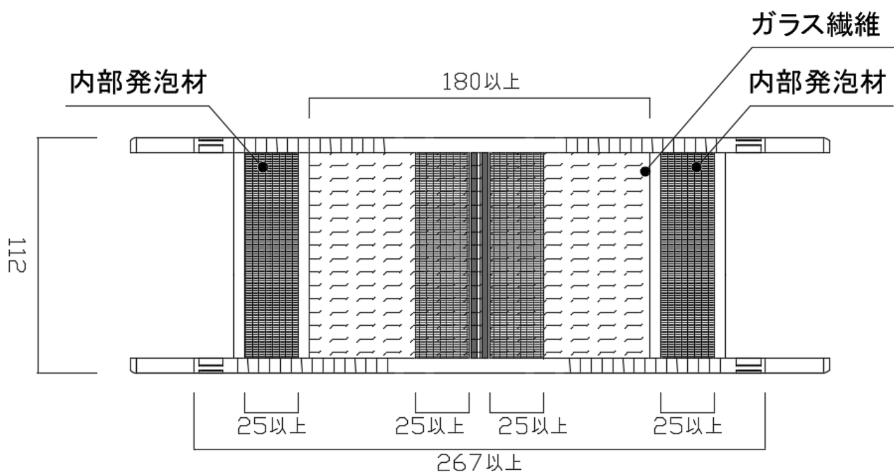
断面図2
